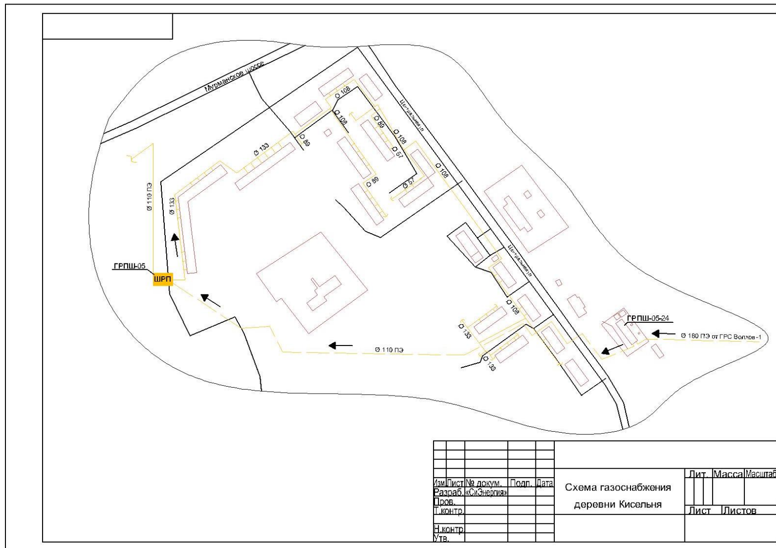
Рисунок 2. Схема газоснабжения д. Кисельня
